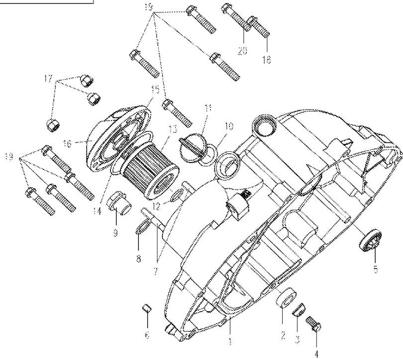
E01-3 右侧盖分总成 RIGHT SIDE COVER
